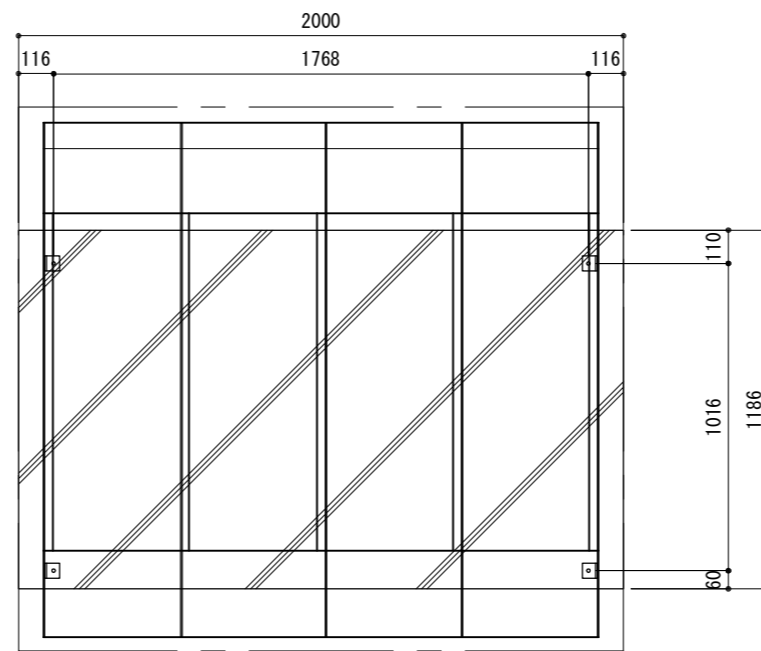
基礎伏図 S = 1 / 25
