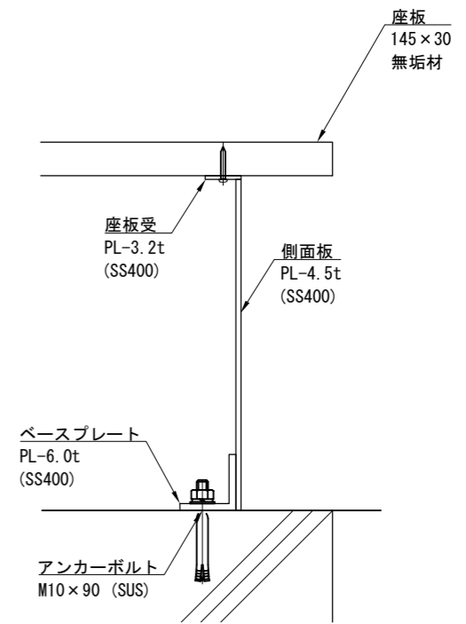
取付詳細図 S = 1 / 6
