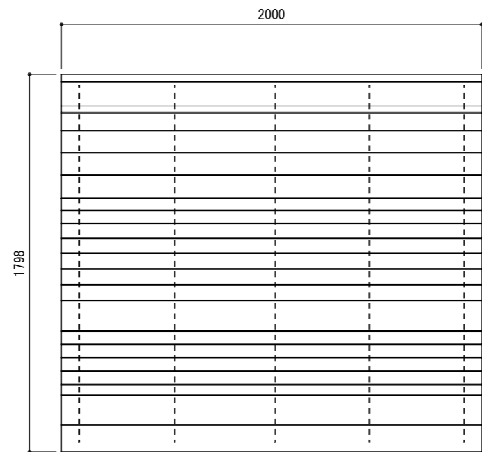
平面図 S = 1 / 25
