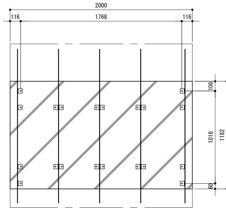
基礎伏図 S=1/25
