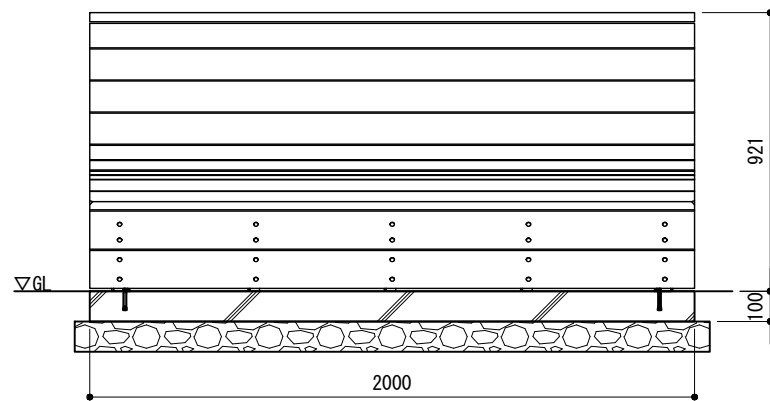
立面図 S=1/25
