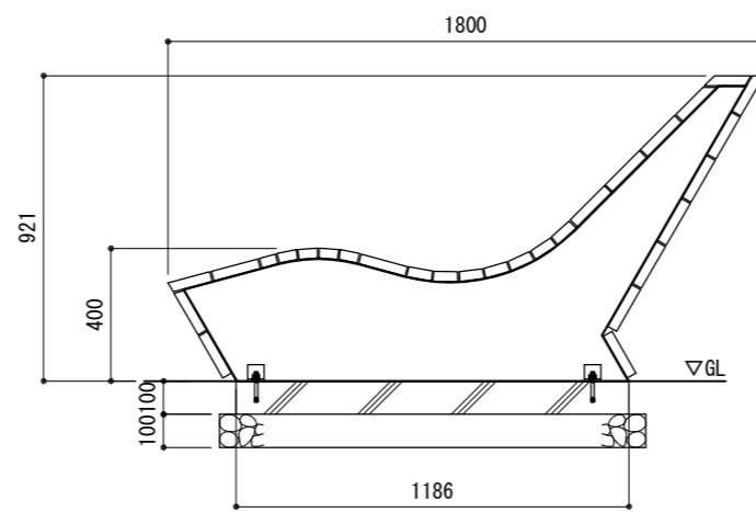
断面図 S = 1 / 25
