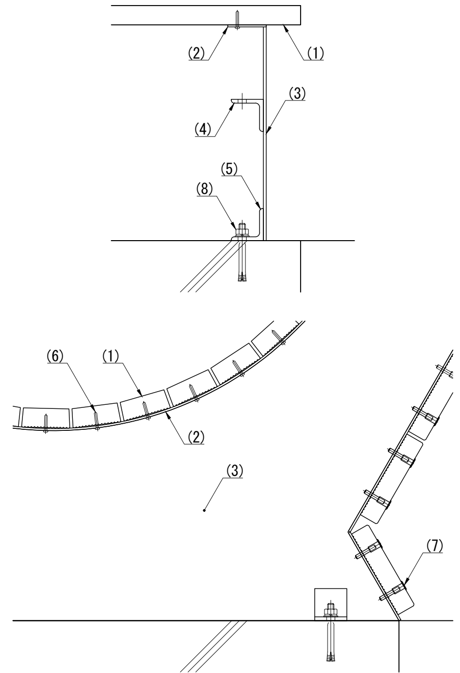
取付詳細図 S=1/6
