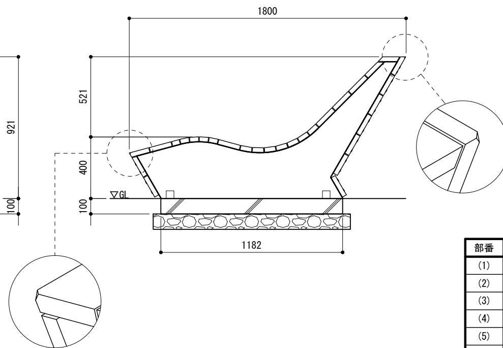
側面図 S=1/25
