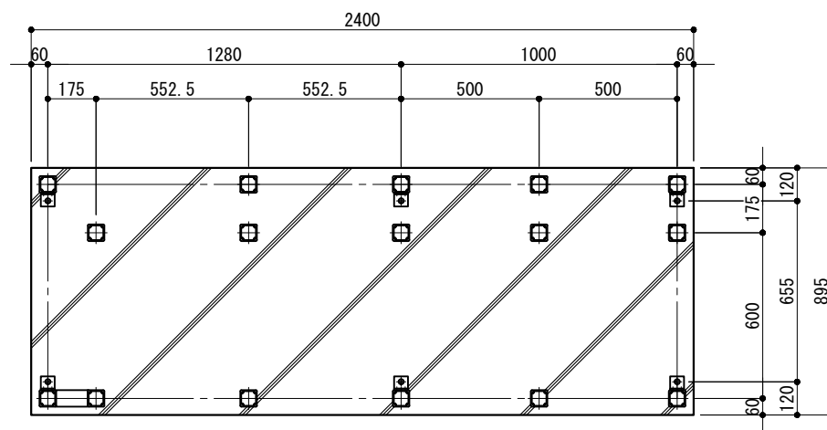
基礎伏図 S=1/25
