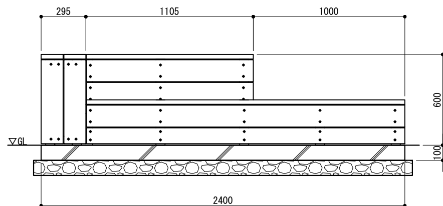
立面図 S=1/25
