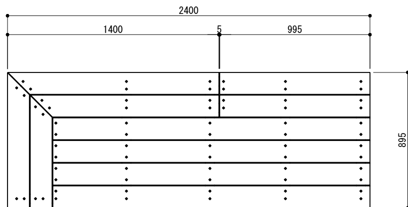
平面図 S=1/25
