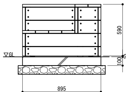
側面図 S=1/25
