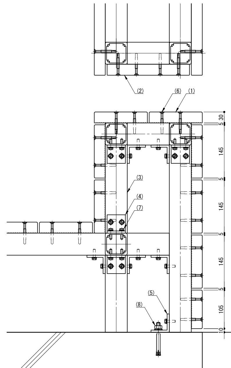
取付詳細図 S=1/6
