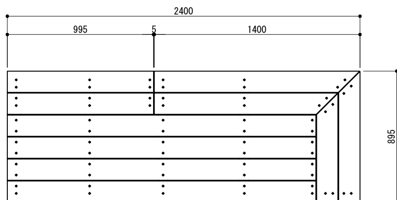
平面図 S=1/25
