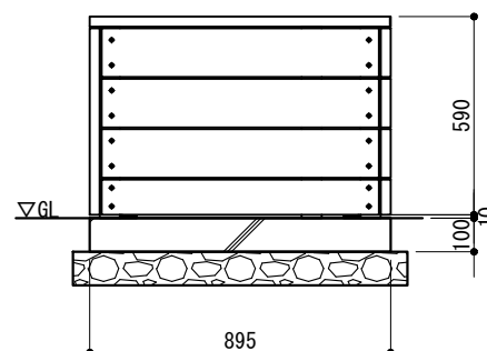
側面図 S=1/25
