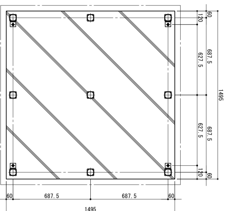
基礎伏図 S=1/20
