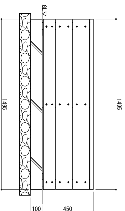
立面図 S=1/20
