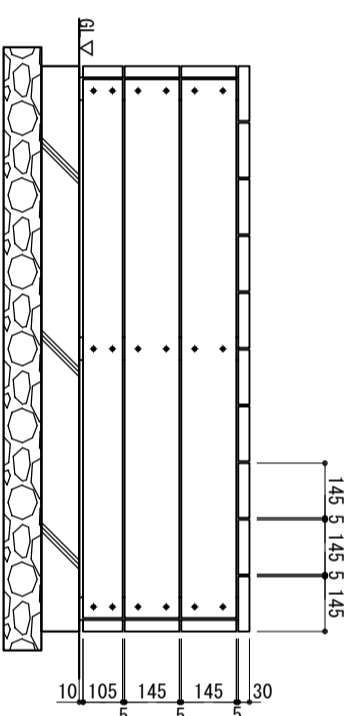
側面図 S=1/20
