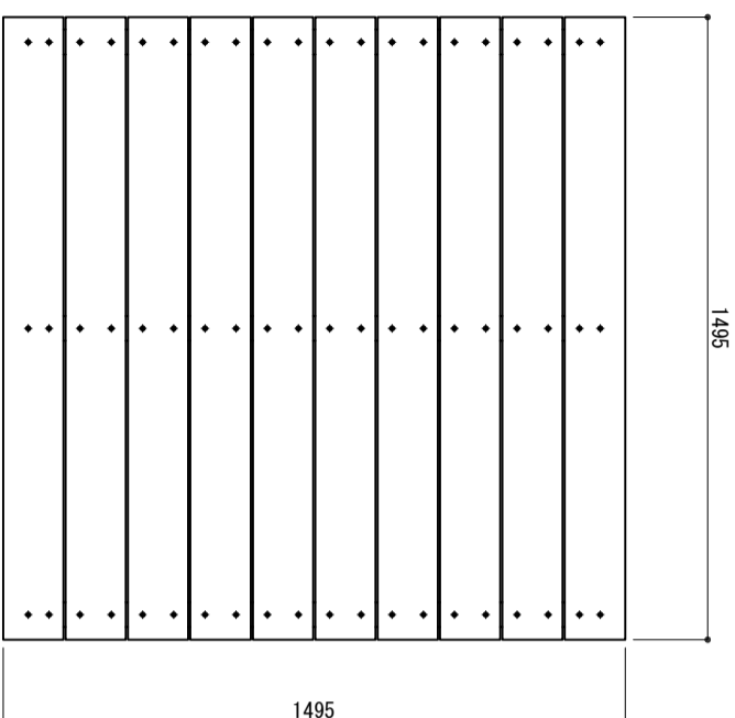
平面図 S=1/20
