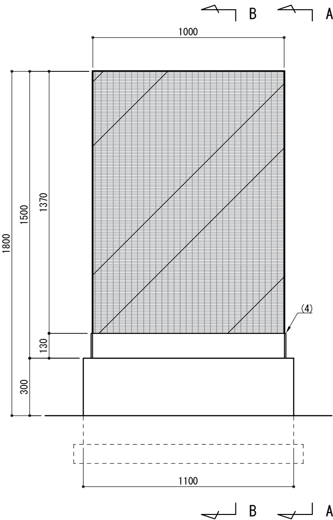
立面図
