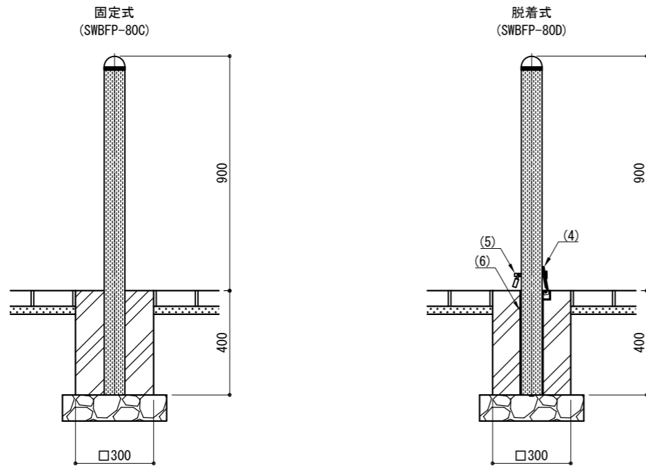
基礎タイプA ◎舗装面に基礎ブロック露出
