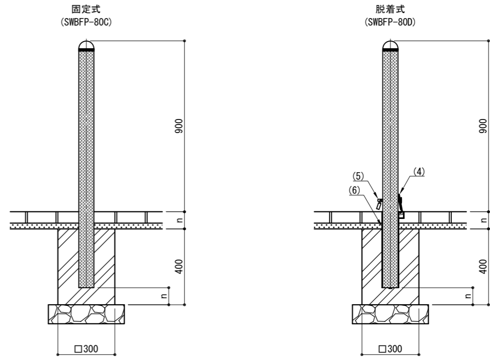
基礎タイプB ◎表面が舗装材
