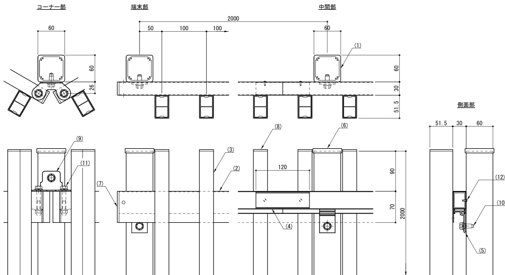
取付詳細図
