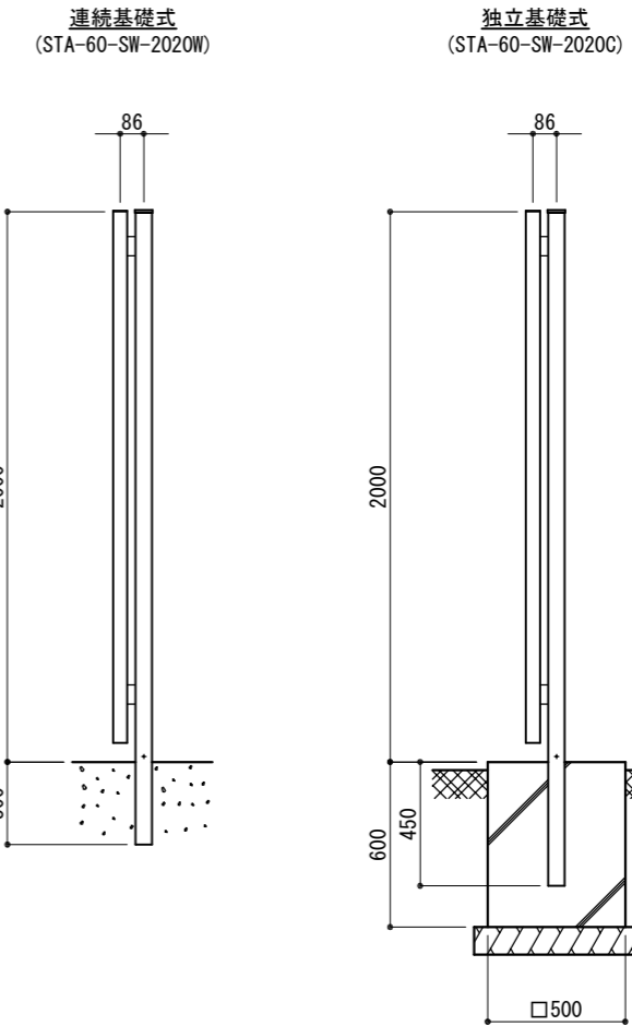
側面図
