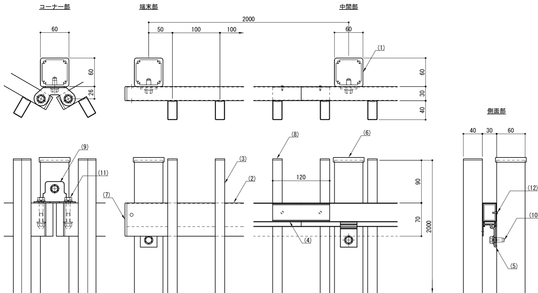
取付詳細図
