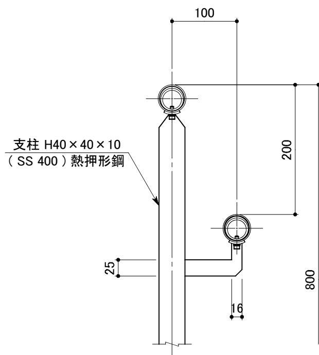
側面図
