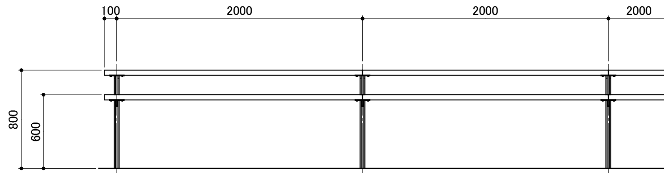
立面図
