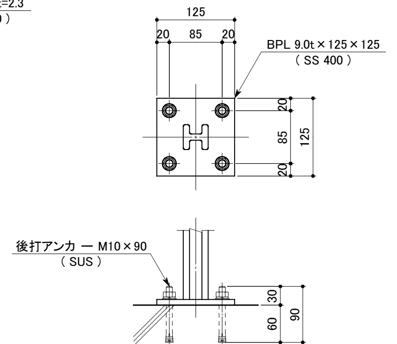
ベース詳細図
