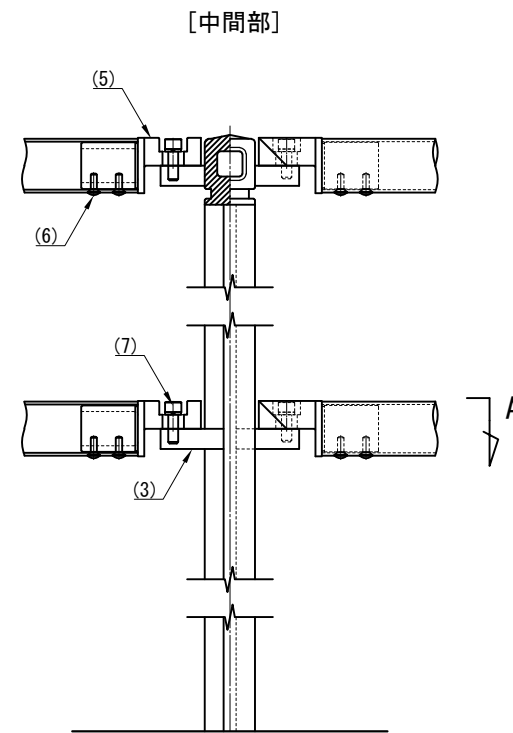
取付詳細図
