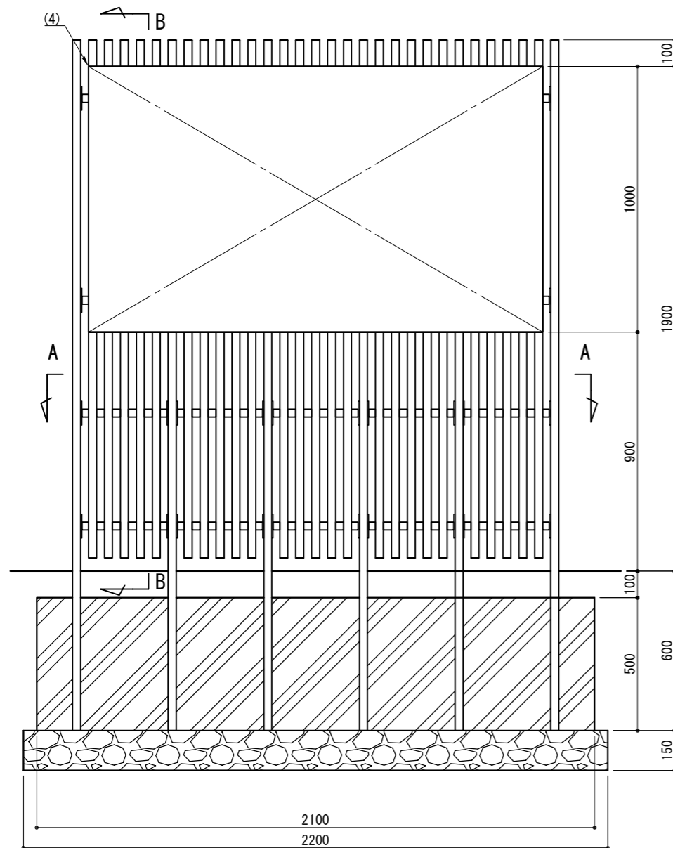
立面図
