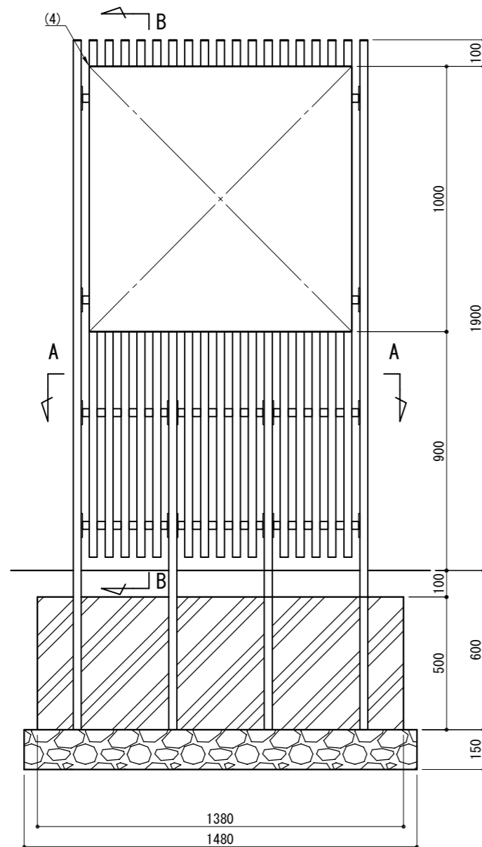
立面図
