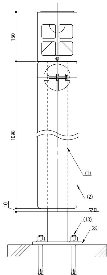
側面図
