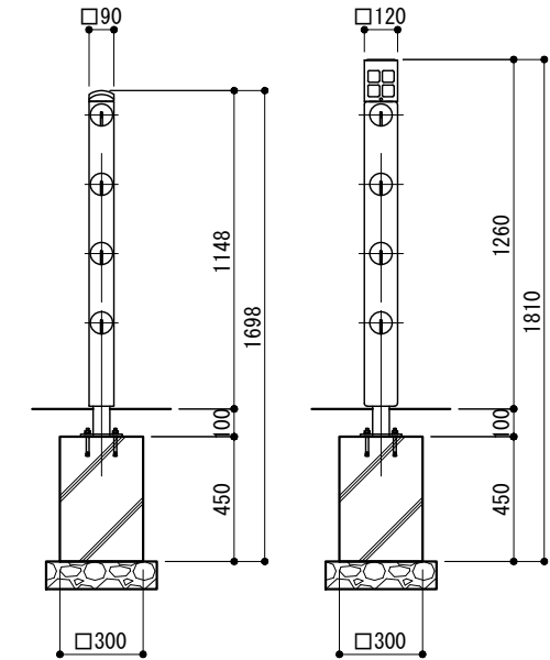
側面図
