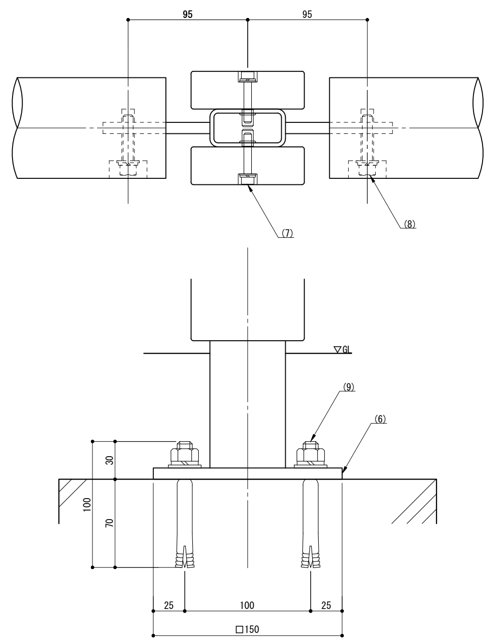
詳細図
