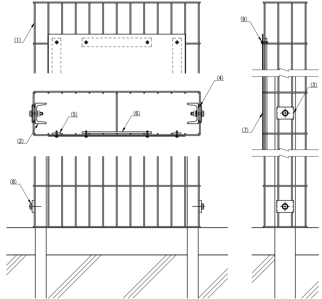
取付詳細図
