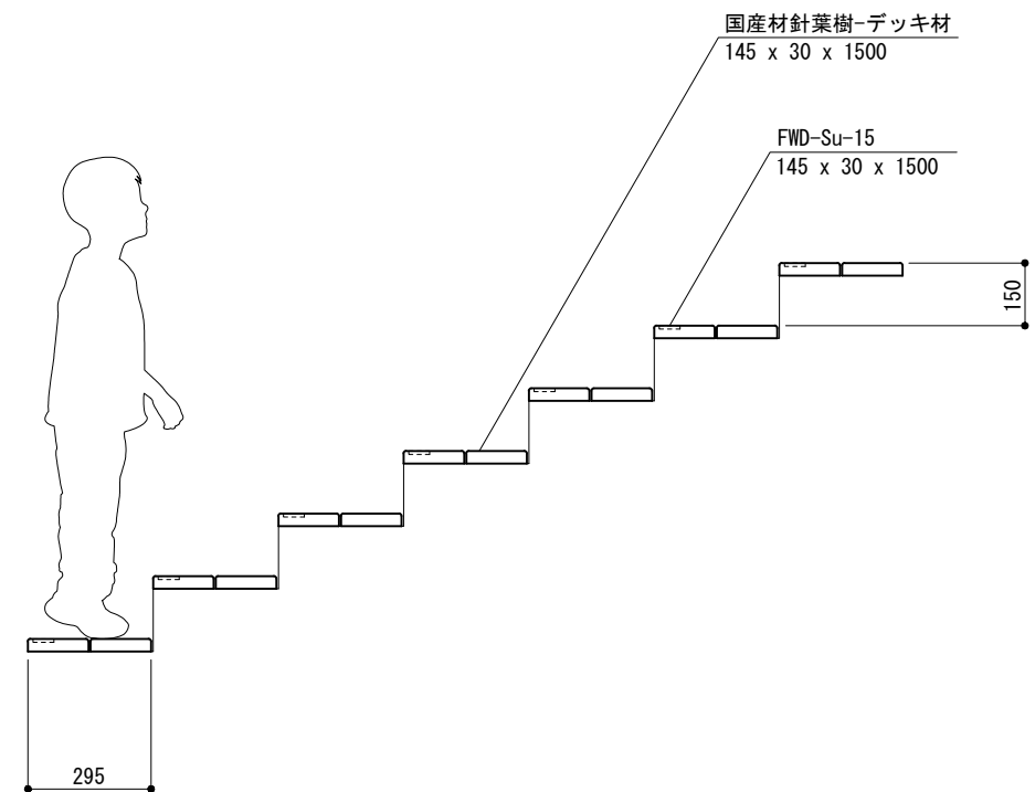
参考取付図 S = 1 : 20
