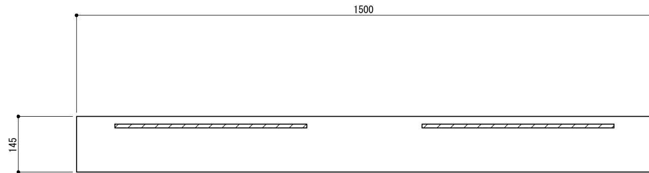
平面図 S = 1 : 10
