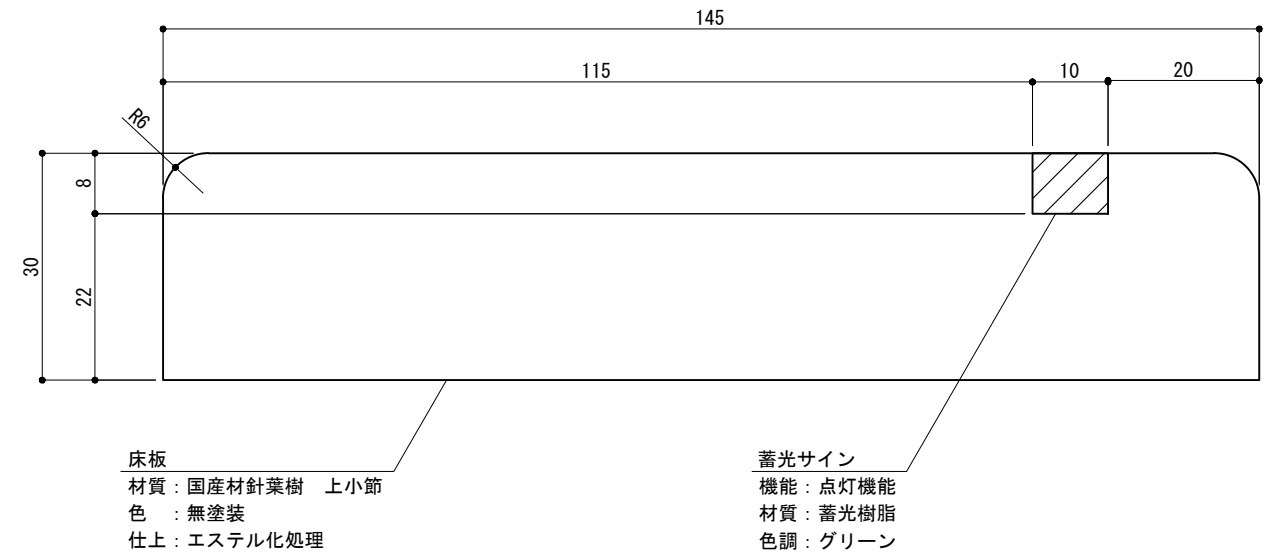
断面図 S = 1 : 1
