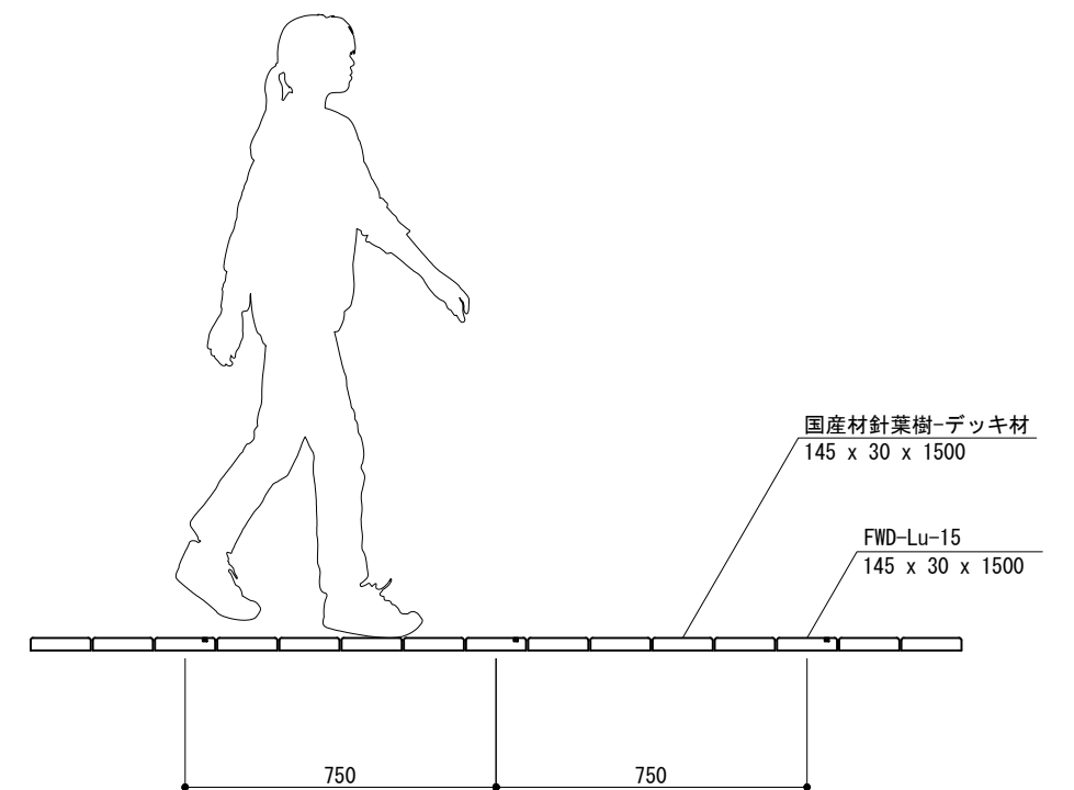
参考取付図 S = 1 : 20
