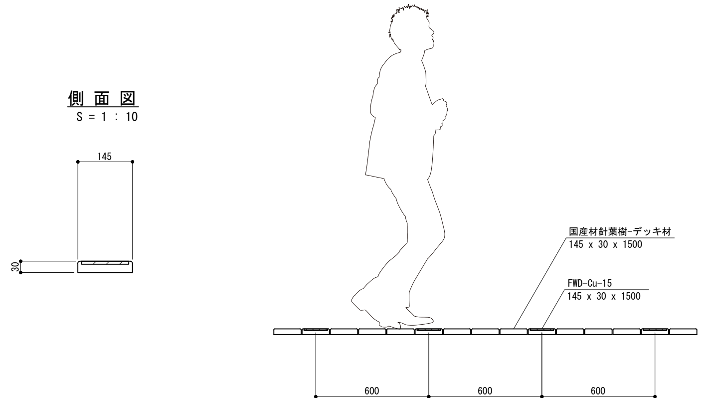
参考取付図 S = 1 : 20
