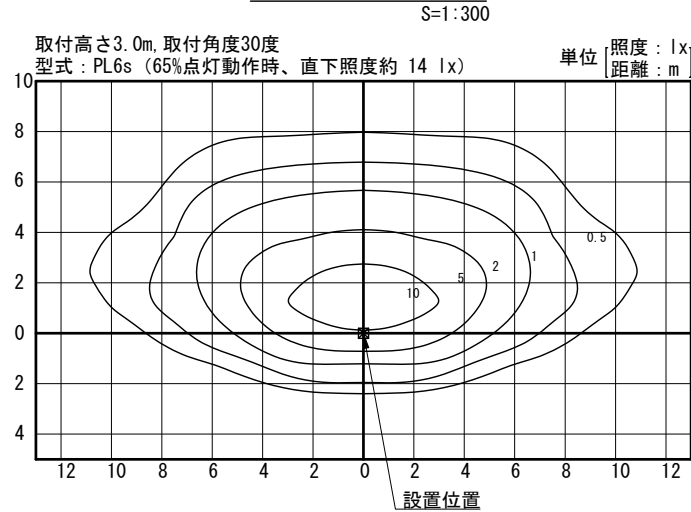
水平面照度分布図
