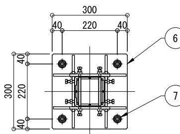
ベース部詳細図 S=1:15
