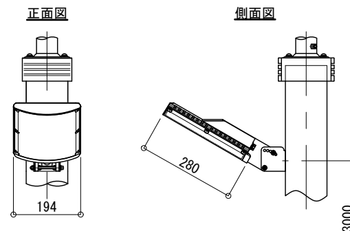
照明器具詳細図 S=1:15
