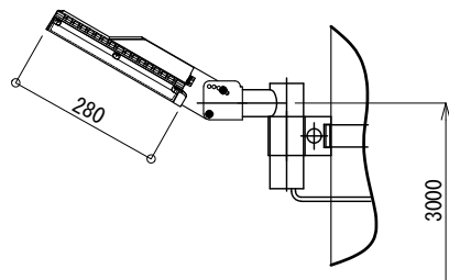
B-B断面図 S=1:15
