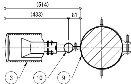
B-B断面図 S=1:15
