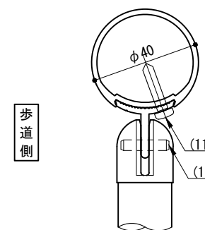
A矢視
