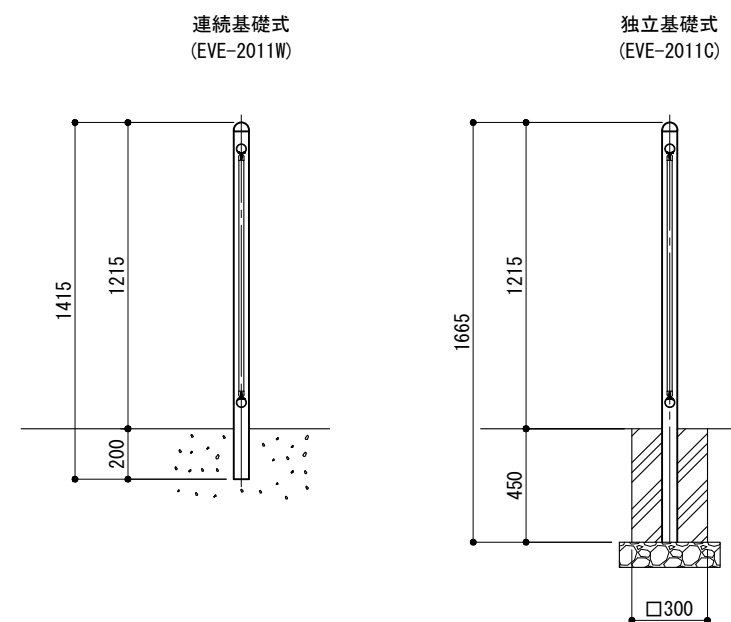
A矢視
