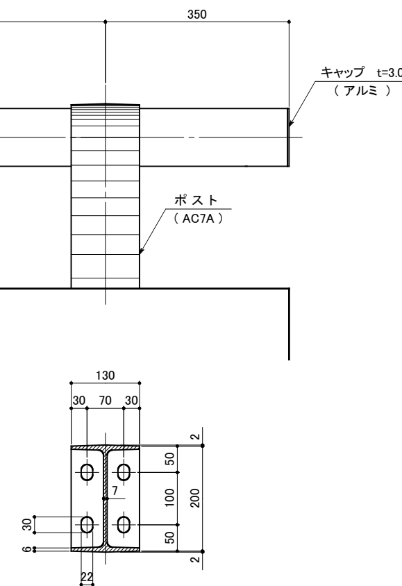
端末部
