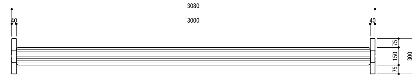
平面図 S=1:20
