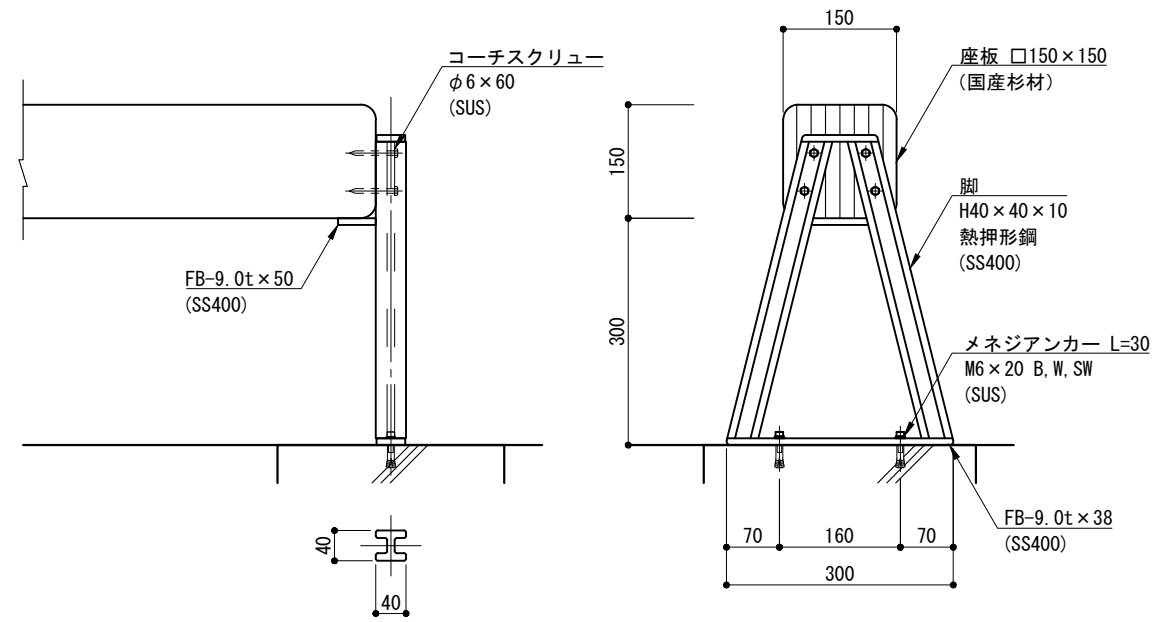
取付詳細図 S=1:10
