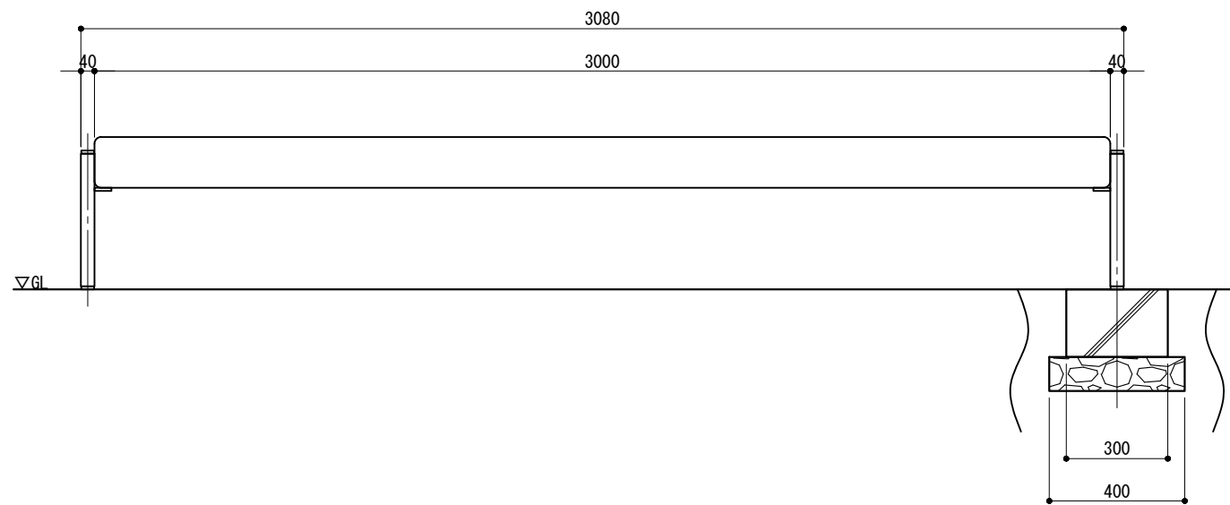
立面図 S=1:20
