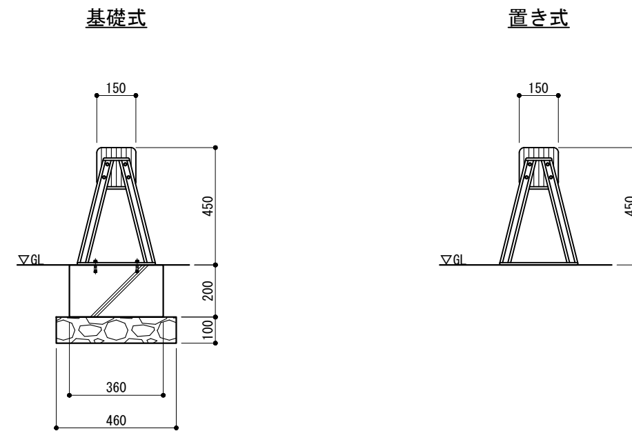
側面図 S=1:20
