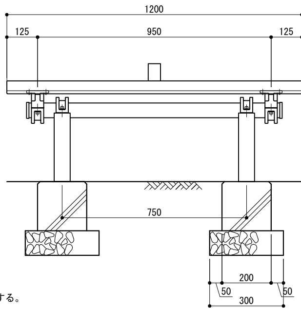
立面図 S = 1 : 15
