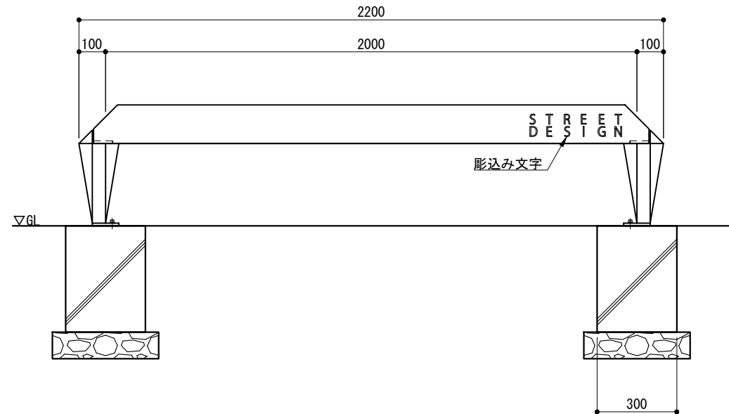
立面図 S=1/20
