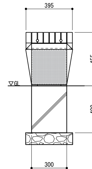
側面図 S=1/20
