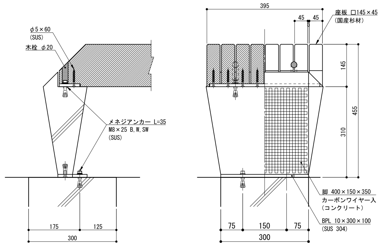
取付詳細図 S=1/8
