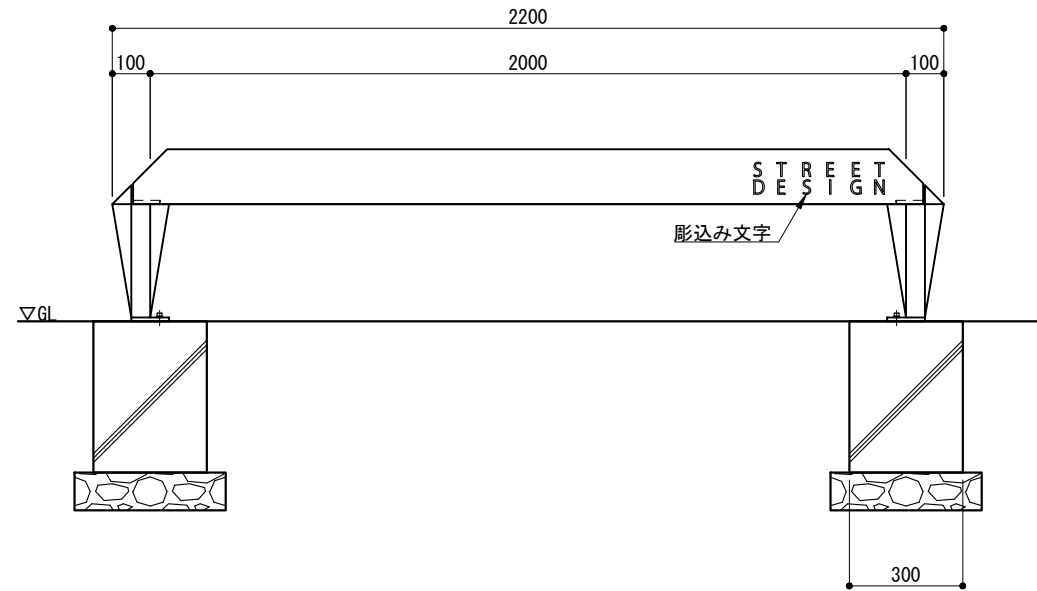
立面図 S=1/20
