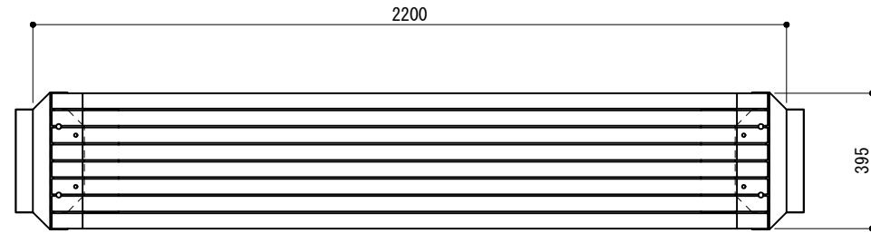
平面図 S=1/20
