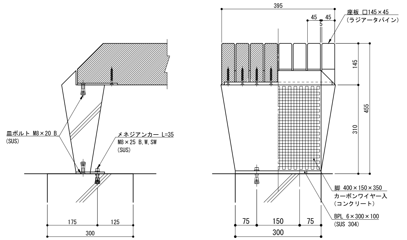
取付詳細図 S=1/8
