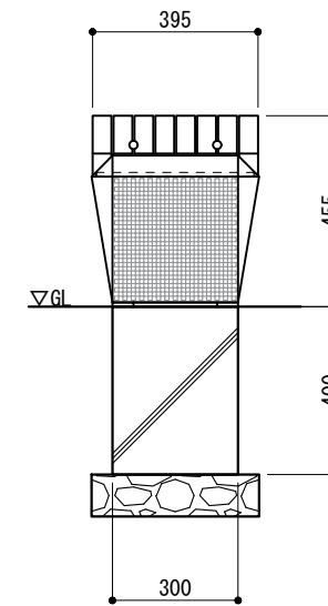
側面図 S=1/20
