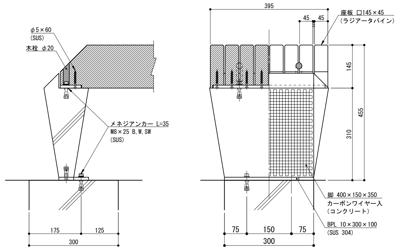
取付詳細図 S=1/8
