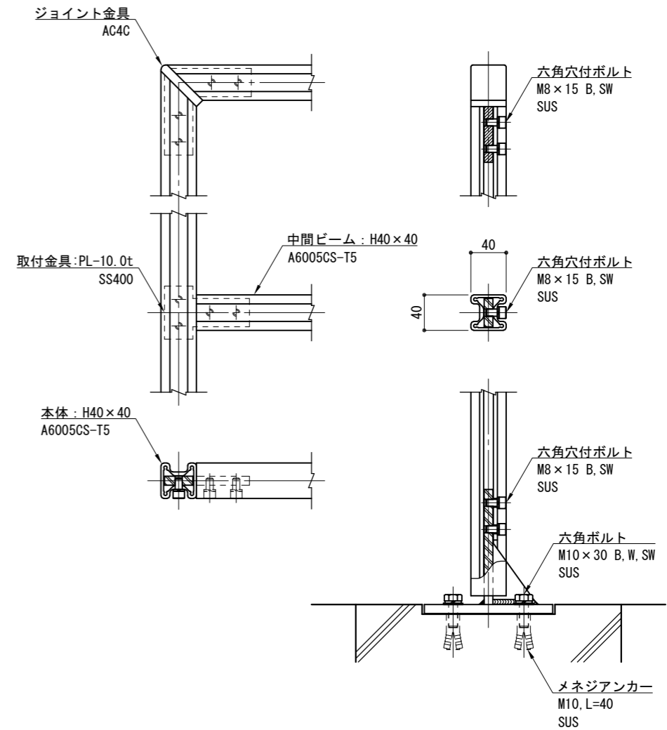
取付詳細図
