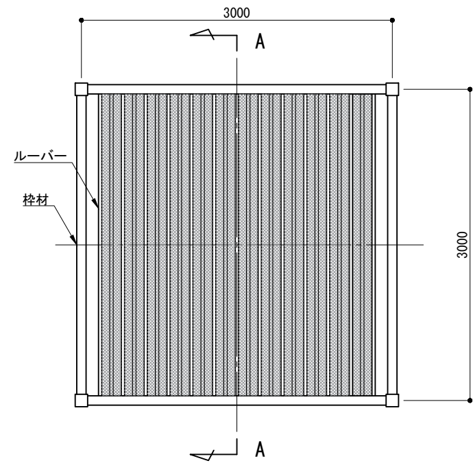
平面図 S=1/50
