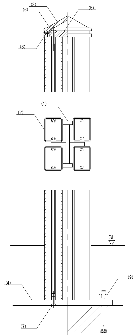
取付詳細図 S = 1 : 3
