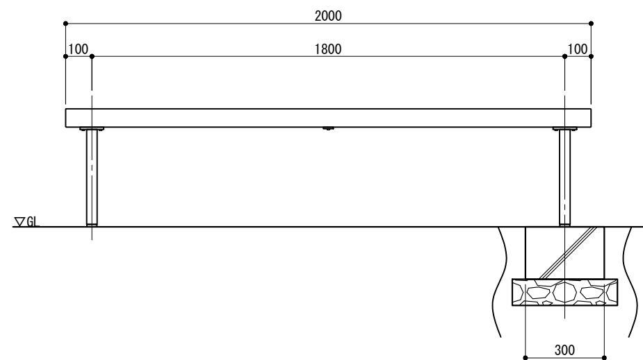
立面図 S=1:20
