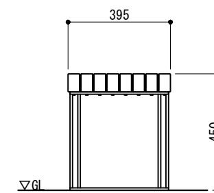
置き式
