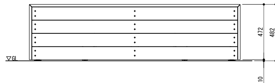
立面図 S=1/20
