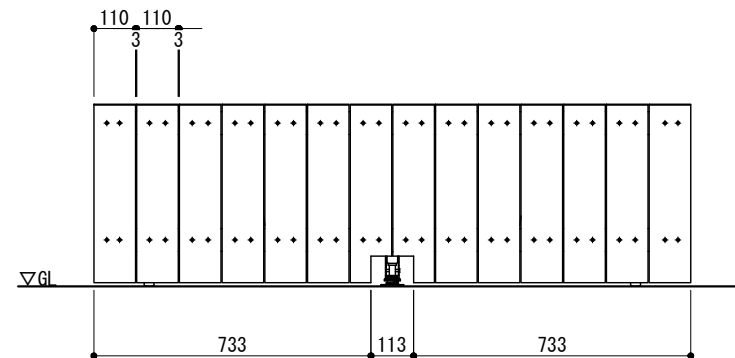
側面図 S=1/20
