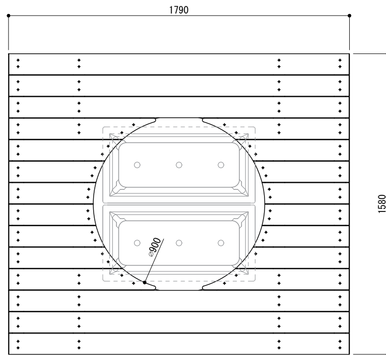
平面図 S=1/20
