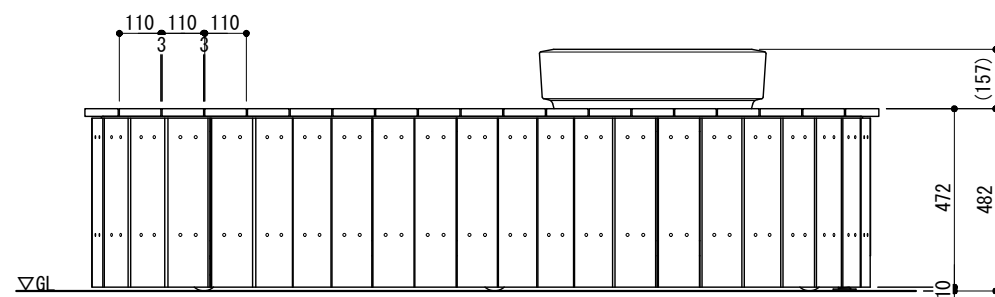
立面図 S=1:20
