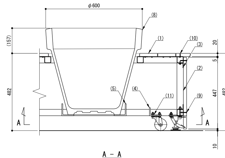
取付詳細図 S=1:12
