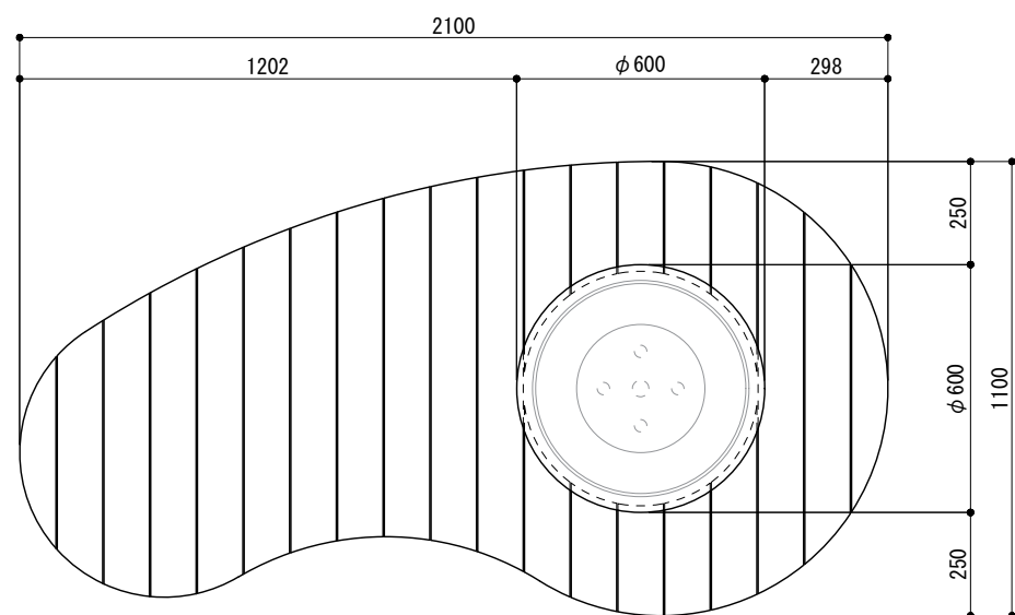
平面図 S=1:20
