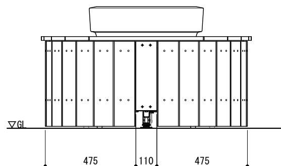
側面図 S=1:20
