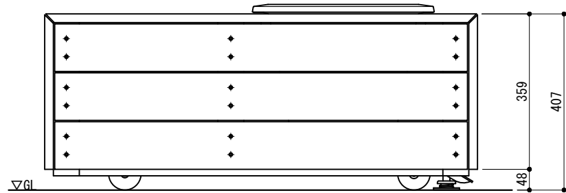
立面図 S=1/12
