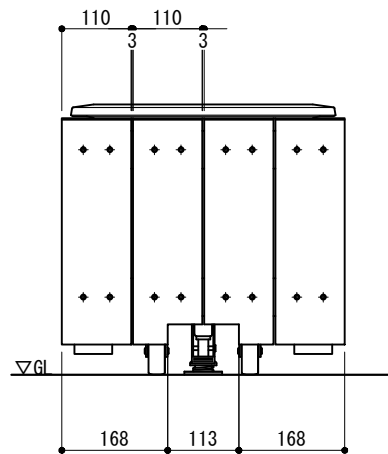
側面図 S=1/12
