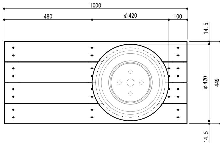
平面図 S=1/12
