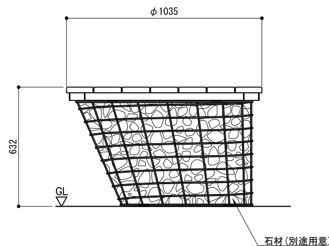
側面図
