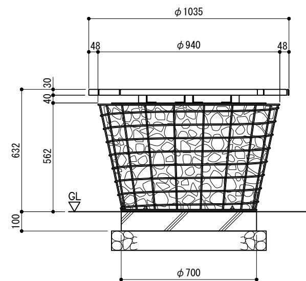
立面図
